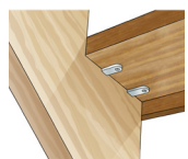
Alt 2. Steginfästning med stegfästjärn
